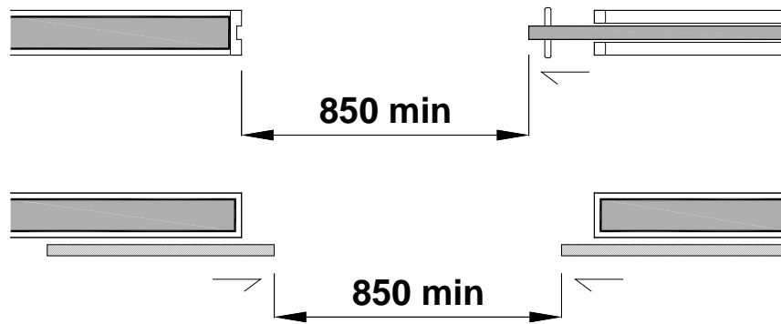
(a) Sliding / automatic door
