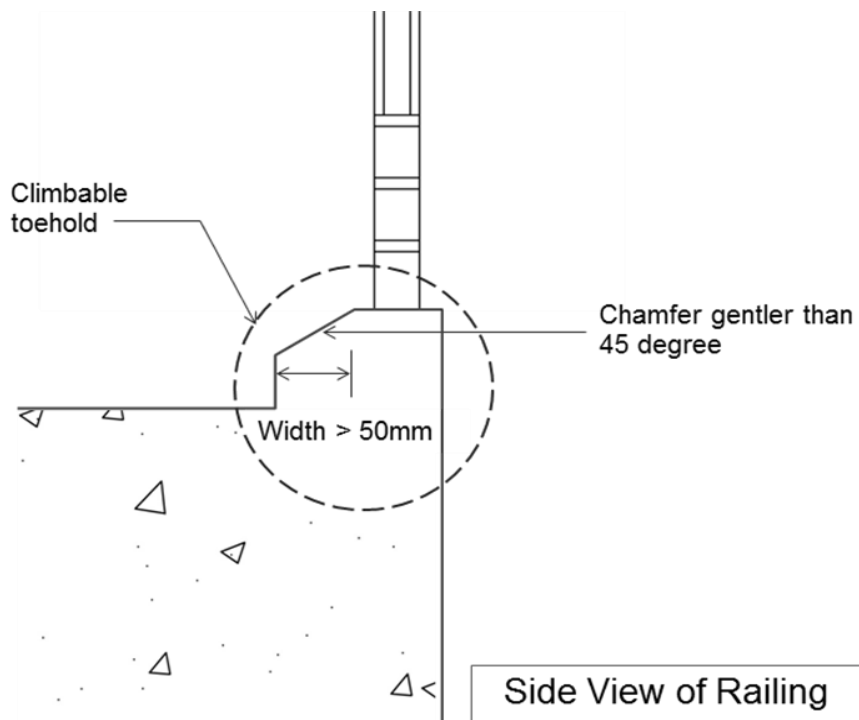
Figure H.3.4A.1(d) – Toehold Dimensions at Kerb/ Protrusion
